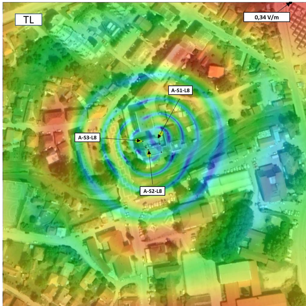
Слика 4.4. Јачина електричног поља на тлу када систем LTE800 оператора А1 Србија ради максималним капацитетом
