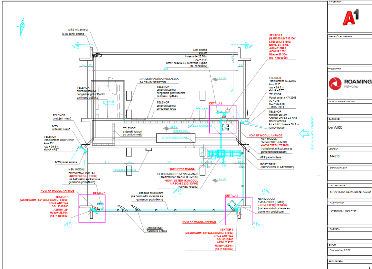
Слика 8.1. Поставни план РБС - основа локације
