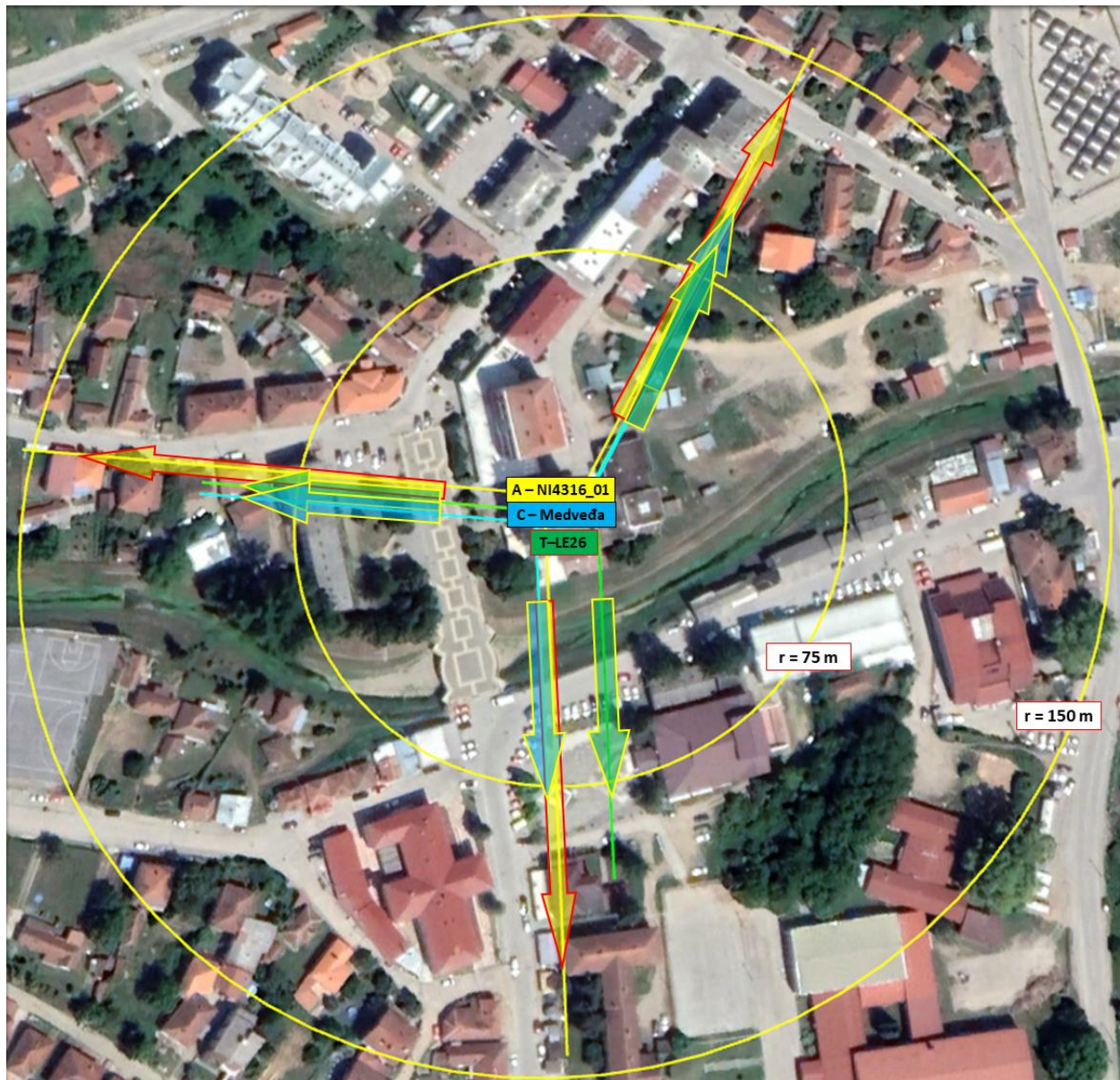
Слика 3.3. Сектори зрачења антена свих извора на локацији
