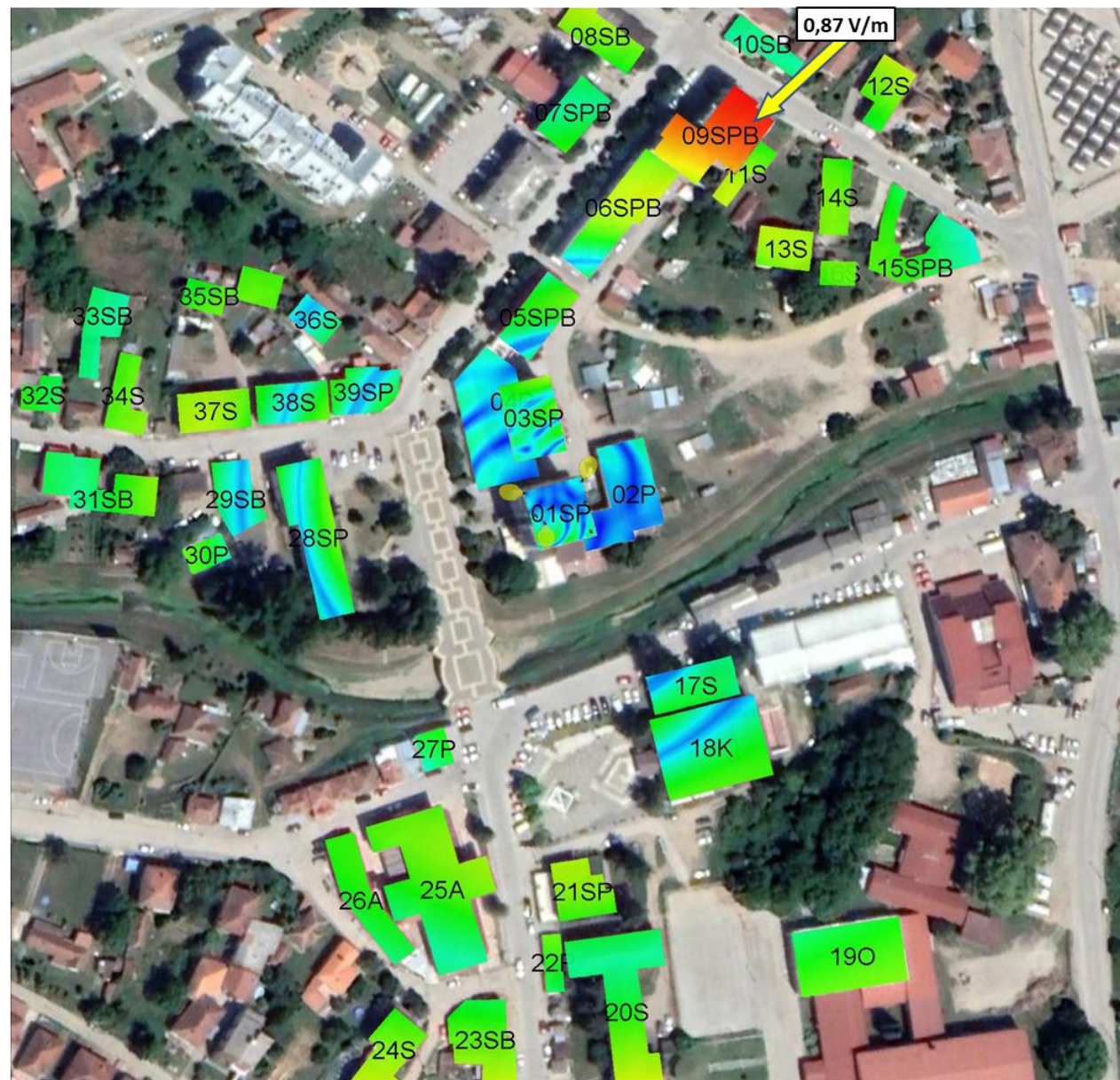
Слика 4.12. Јачина електричног поља унутар објекта када систем LTE1800 оператора А1 Србија ради максималним капацитетом
