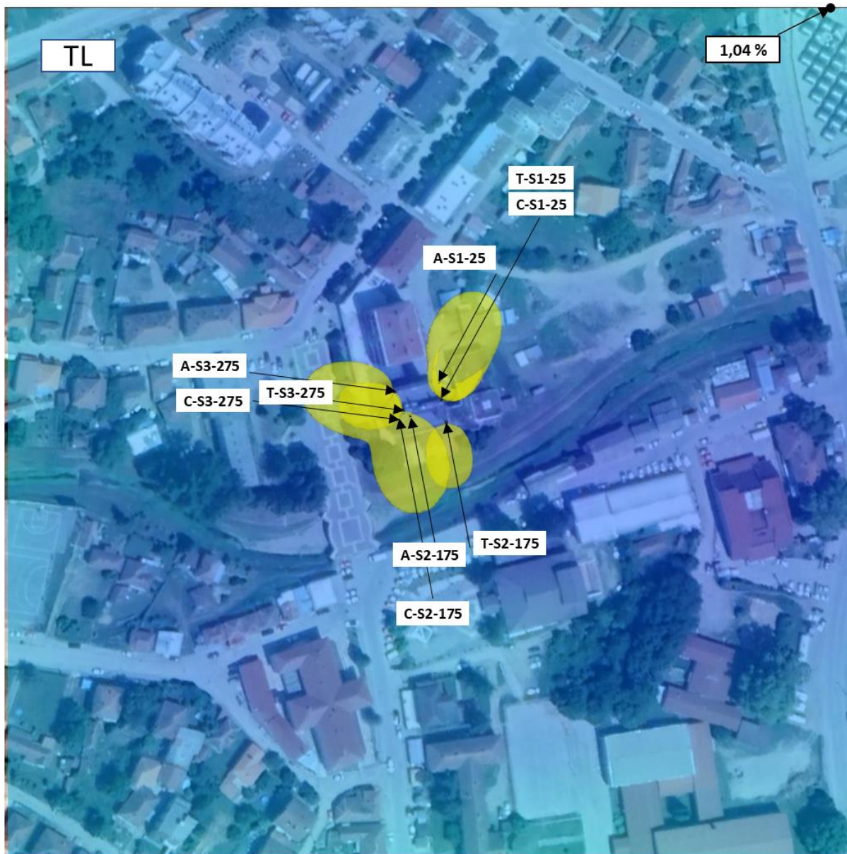
Слика 4.8. Фактор изложености на тлу када сви системи свих оператора раде максималним капацитетом
