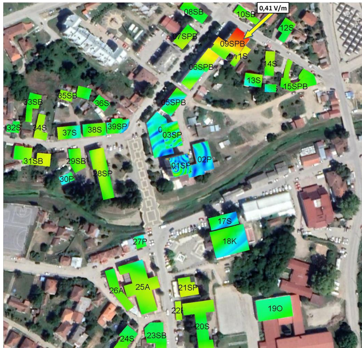
Слика 4.13. Јачина електричног поља унутар објекта када систем LTE2100 оператора А1 Србија ради максималним капацитетом
