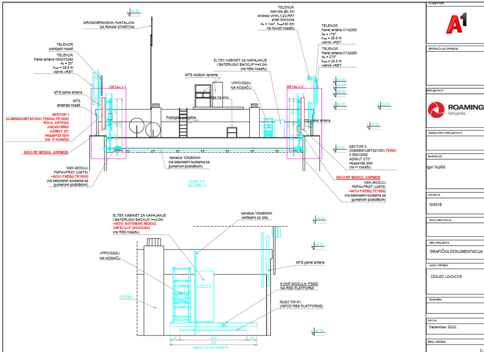
Слика 8.2. Поставни план РБС - изглед локације
