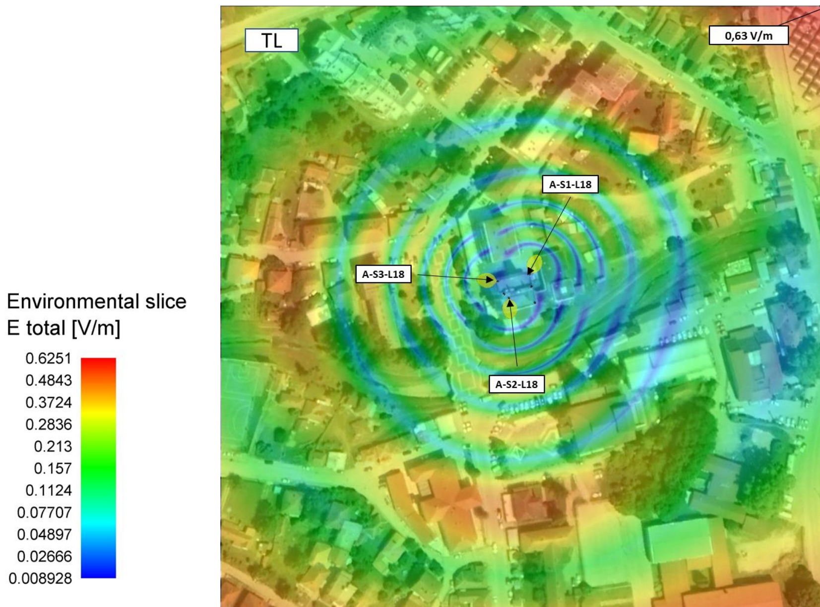
Слика 4.5. Јачина електричног поља на тлу када систем LTE1800 оператора А1 Србија ради максималним капацитетом
