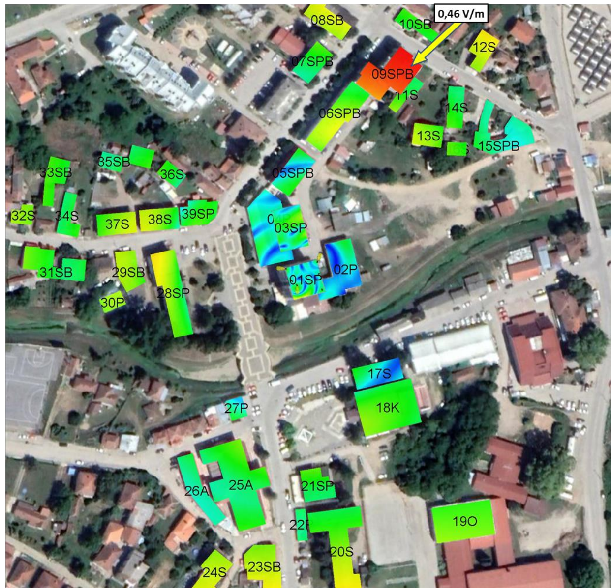
Слика 4.11. Јачина електричног поља унутар објеката када систем LTE800 оператора А1 Србија ради максималним капацитетом
