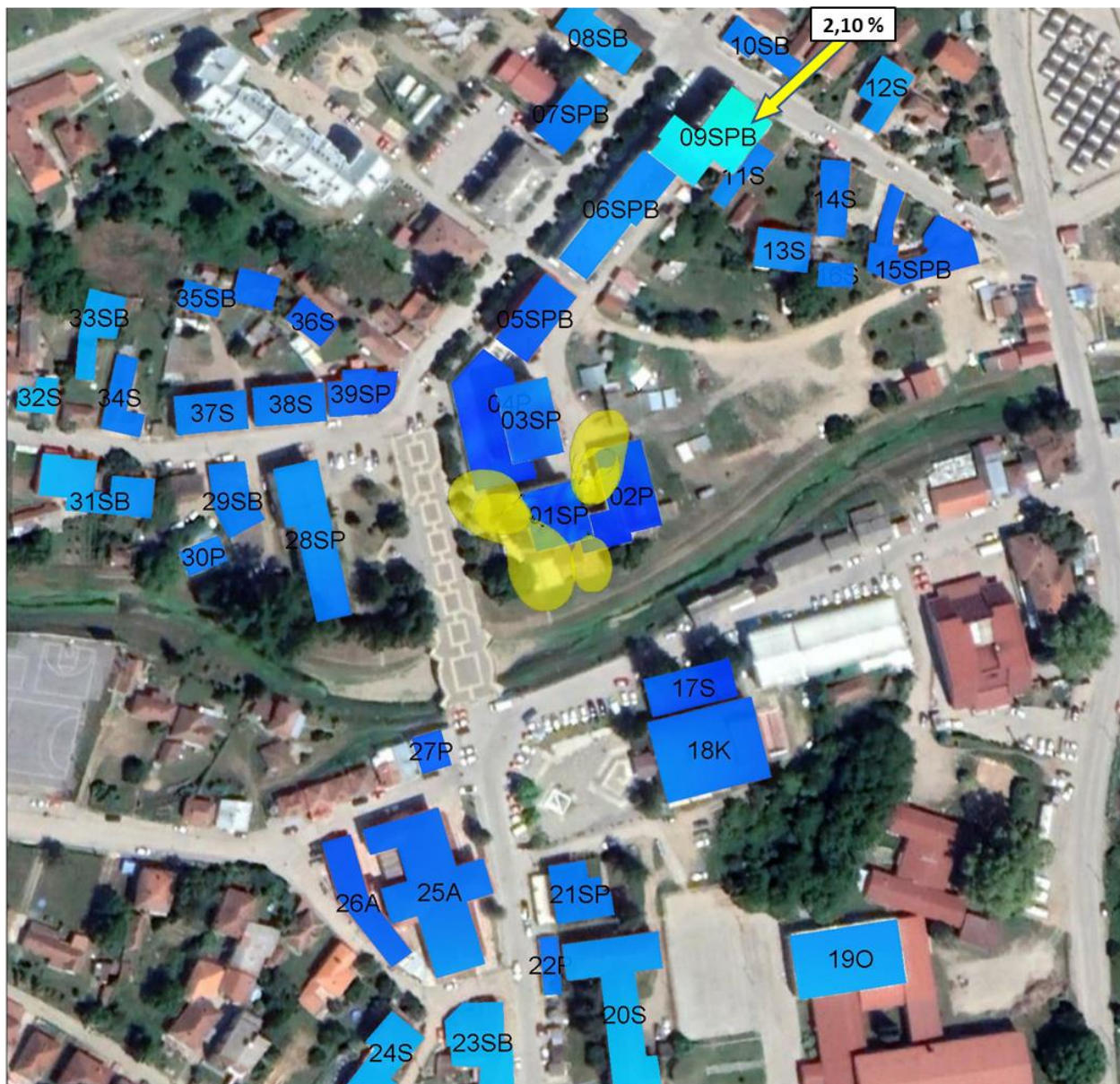
Слика 4.15. Фактор изложености унутар објеката када сви системи свих оператора раде максималним капацитетом
