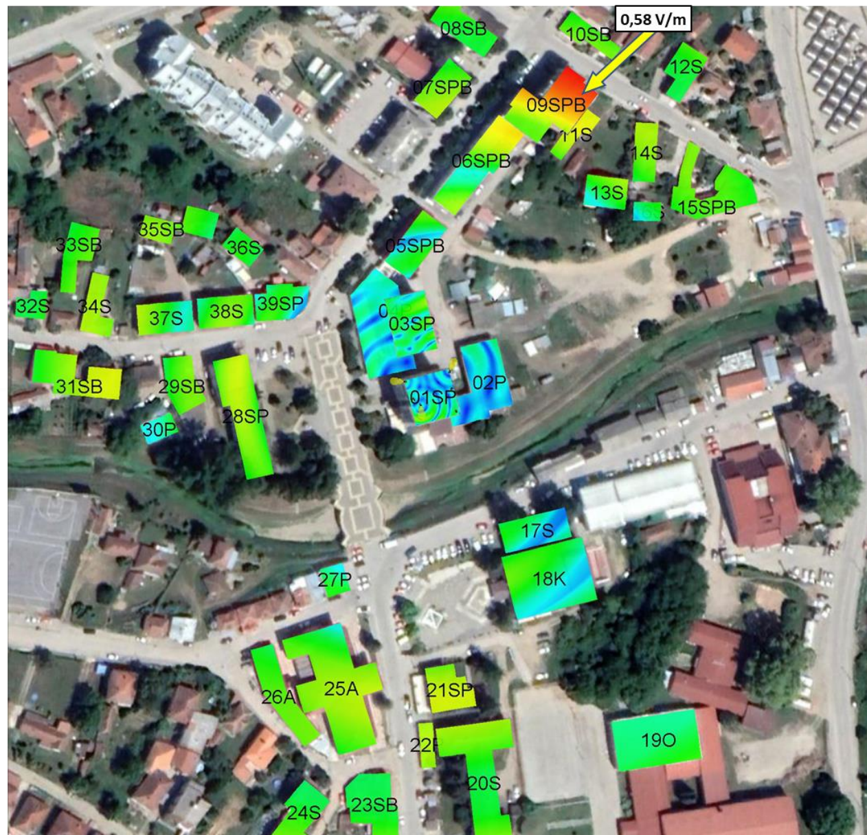
Слика 4.10. Јачина електричног поља унутар објекта када систем UMTS2100 оператора А1 Србија ради максималним капацитетом
