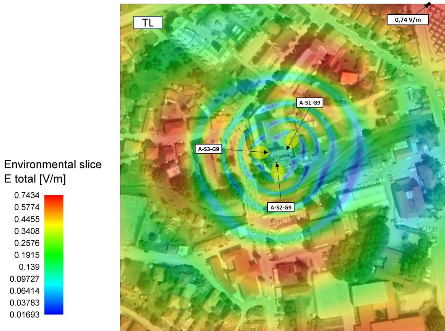
Слика 4.2. Јачина електричног поља на тлу када систем GSM900 оператора А1 Србија ради максималним капацитетом
