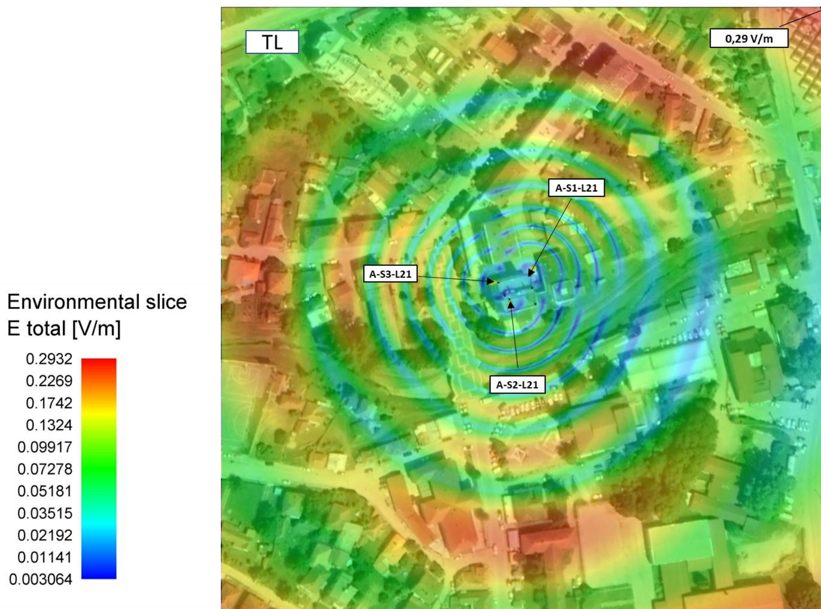
Слика 4.6. Јачина електричног поља на тлу када систем LTE2100 оператора А1 Србија ради максималним капацитетом
