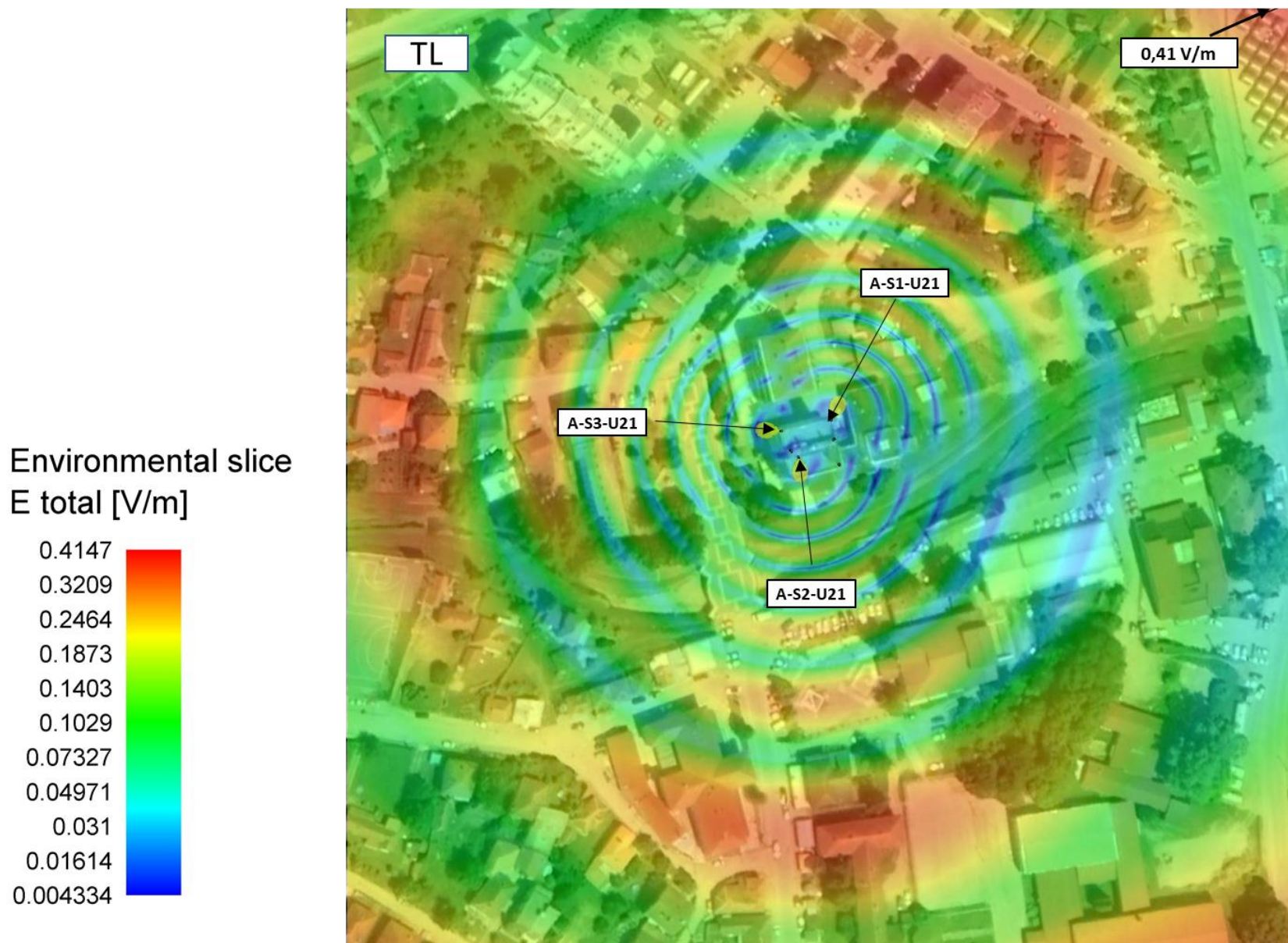
Слика 4.3. Јачина електричног поља на тлу када систем UMTS2100 оператора А1 Србија ради максималним капацитетом
